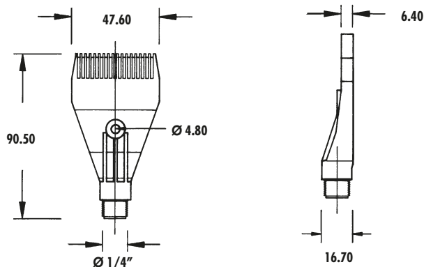
Tipo - 727PP - Type
