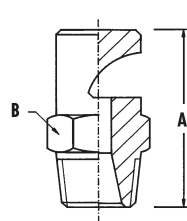
Componenti serie - RL - Series components
