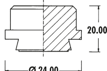
Tappo R2CR Plug
