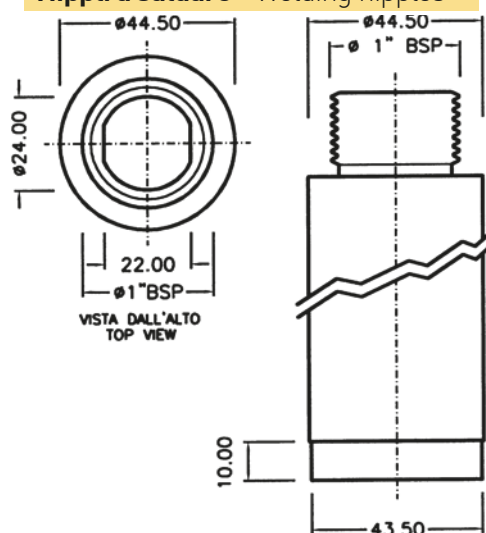
Nippli a saldare - Welding nipples
